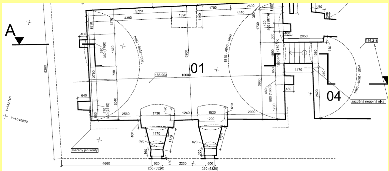
Obrázek 1: Část půdorysu suterénu
