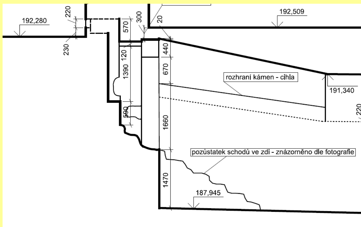
Obrázek 2: Část řezu B - B'
