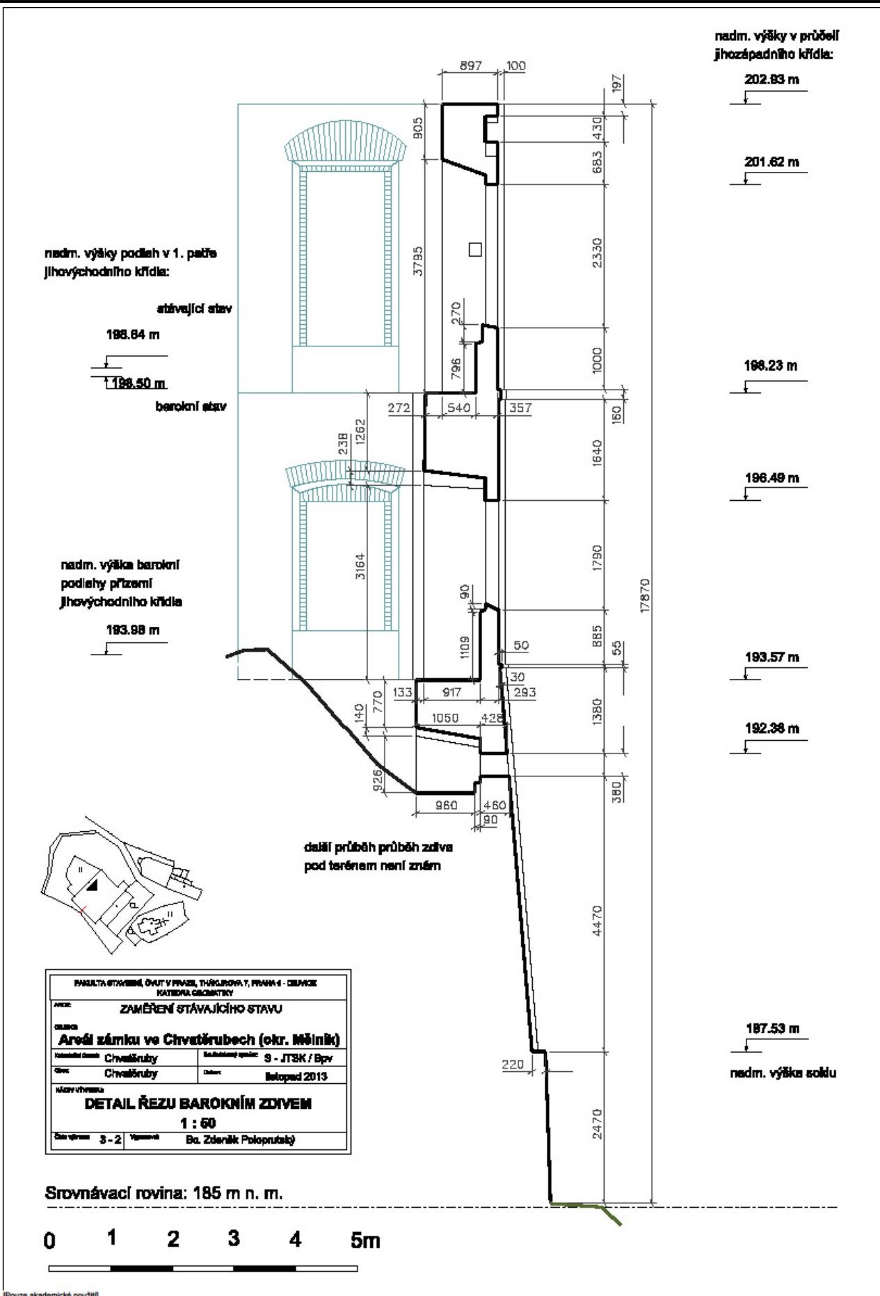
Obr. 1: Detail řezu barokním zdivem
