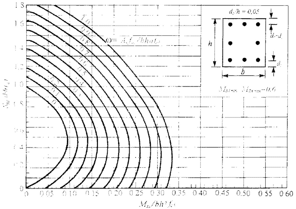
Nomogram 12.14
