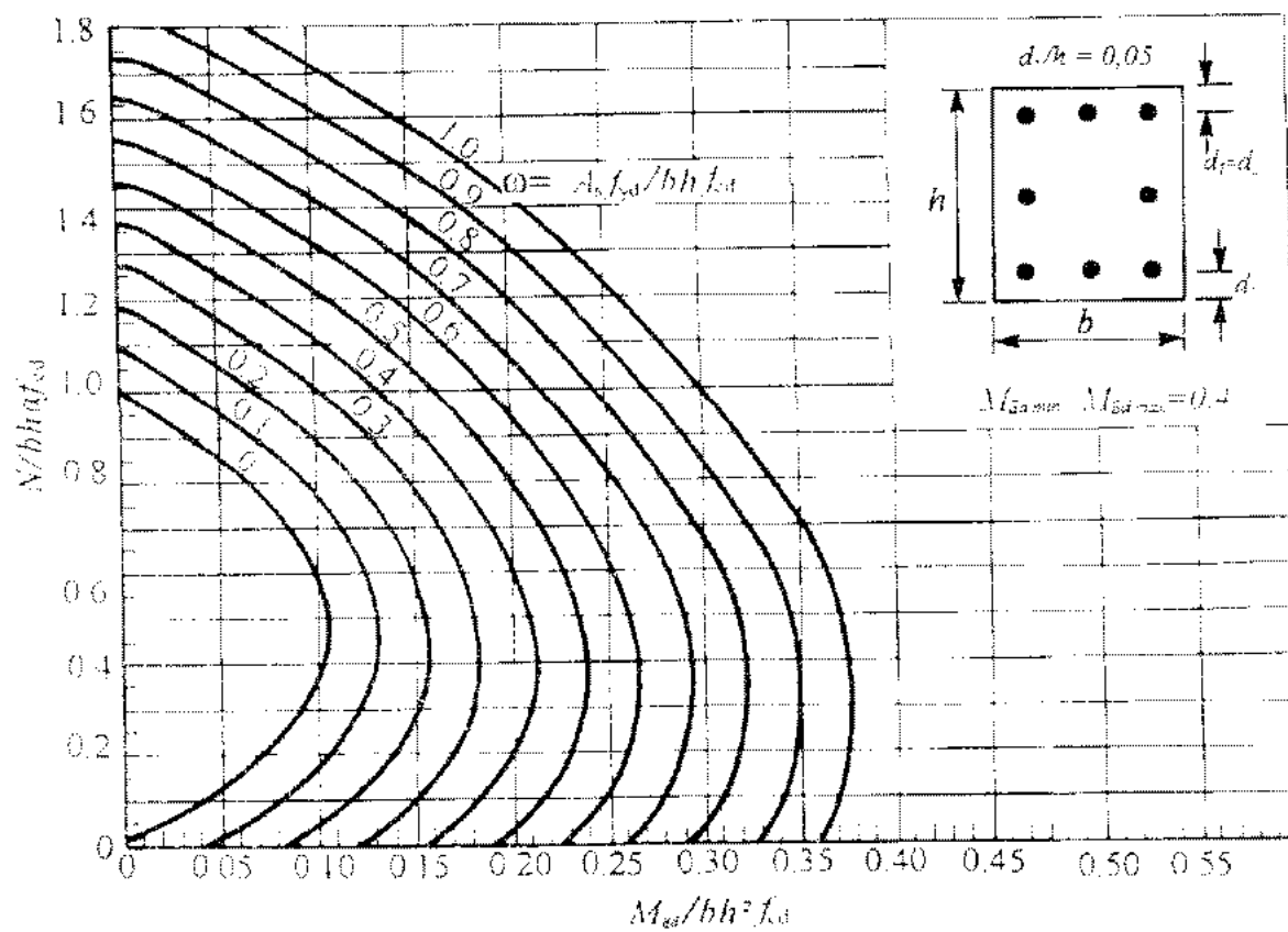
Nomogram 12.12
