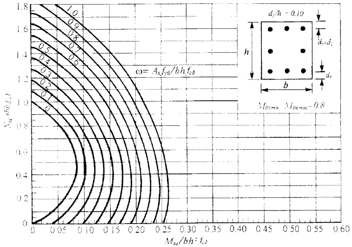
Nomogram 12.20
