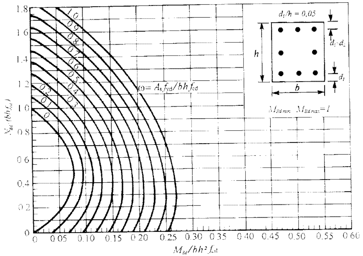
Nomogram 12.16
