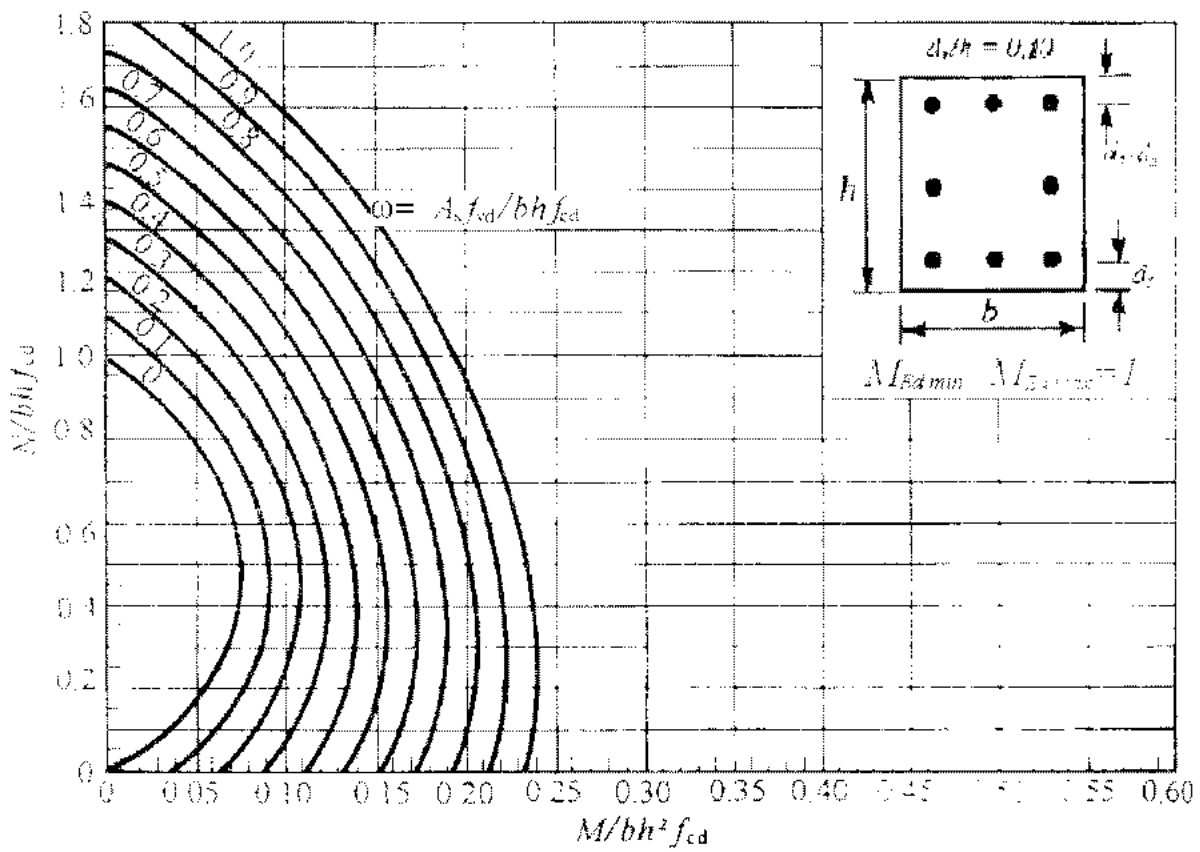
Nomogram 12.20
