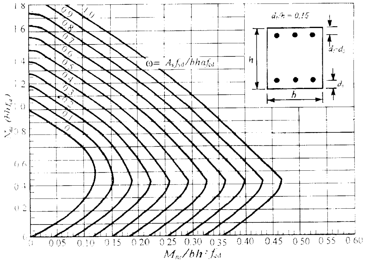
Nomogram 12.4
