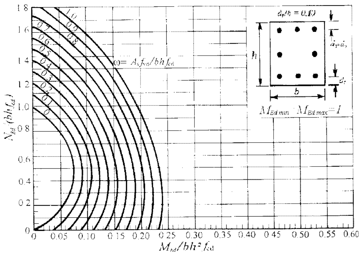
Nomogram 12.16
