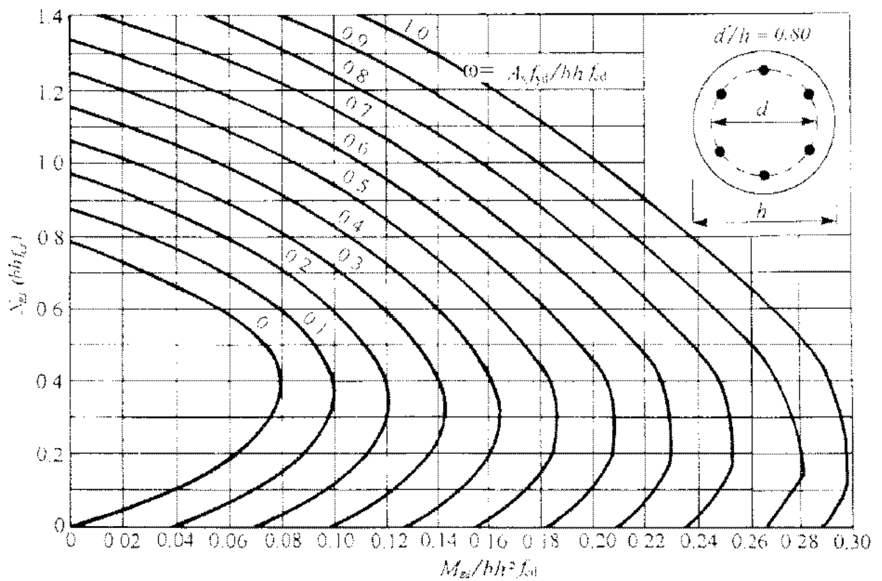
Nomogram 12.8
