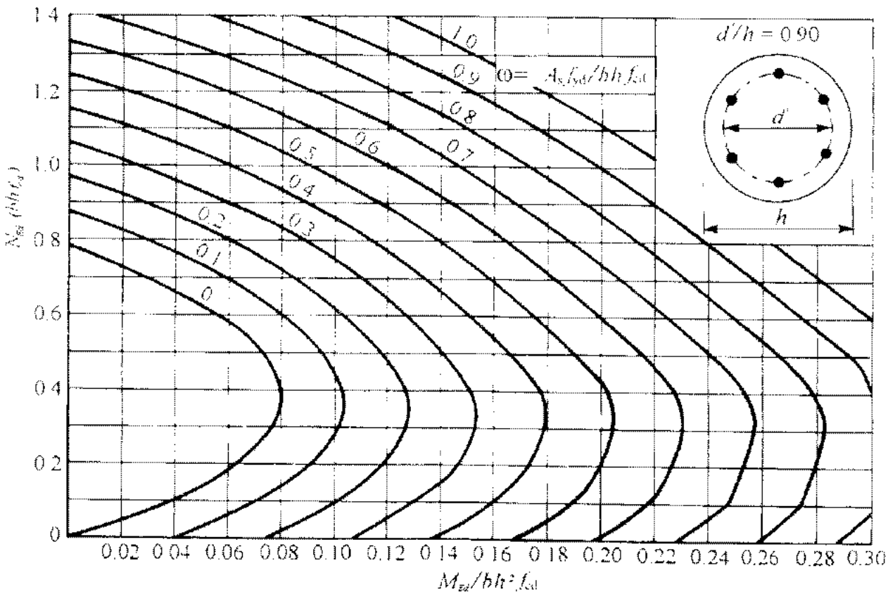
Nomogram 12.10
