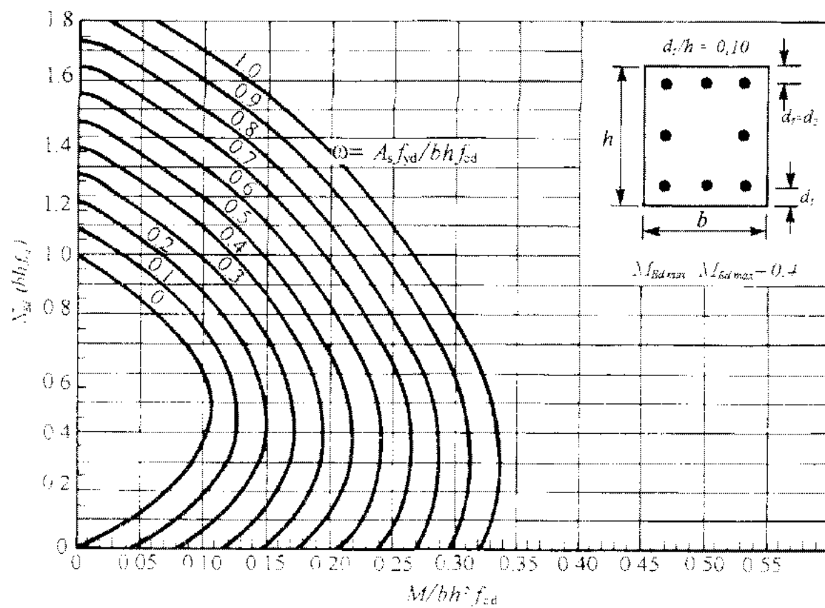
Nomogram 12.18
