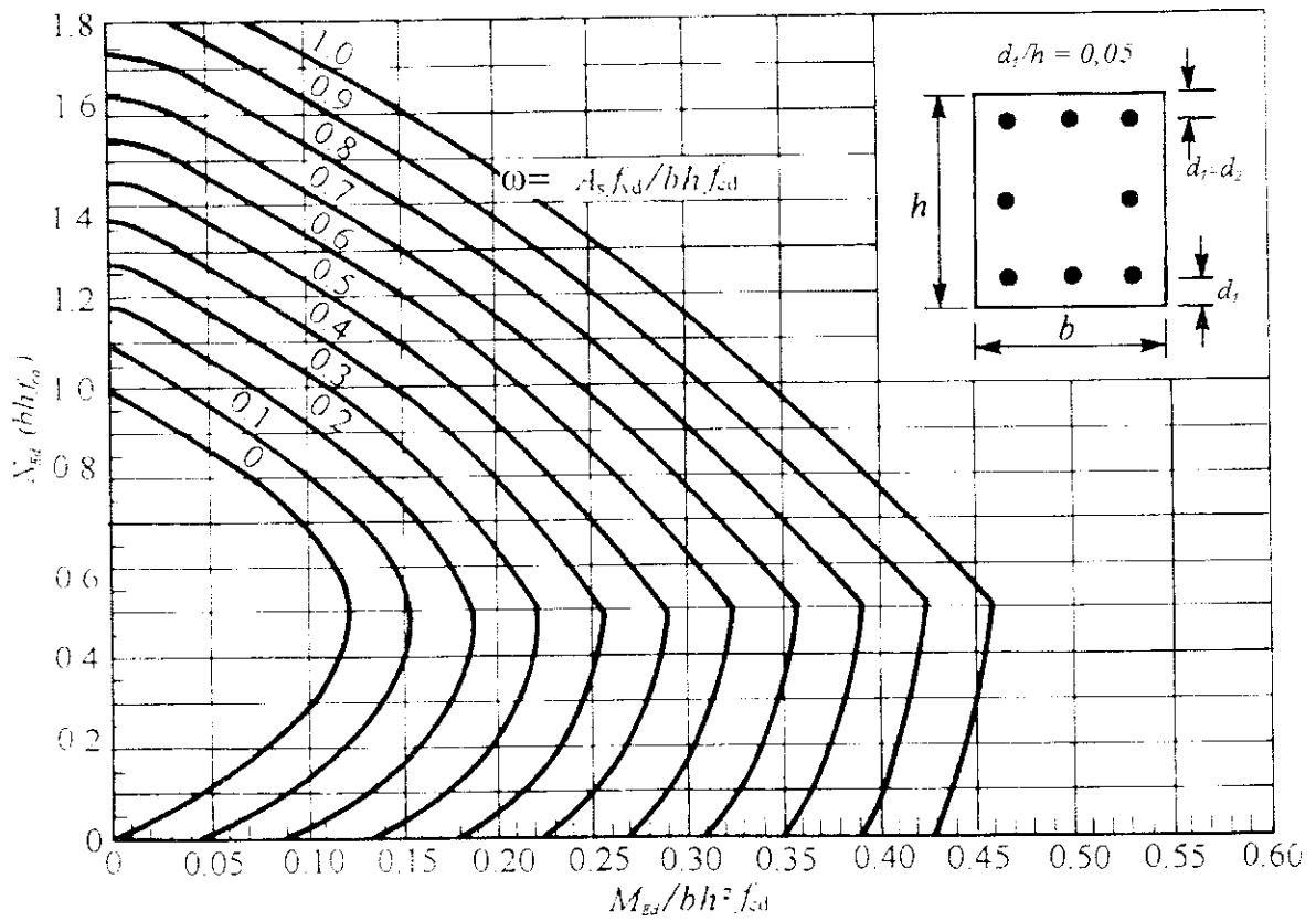
Nomogram 12.4
