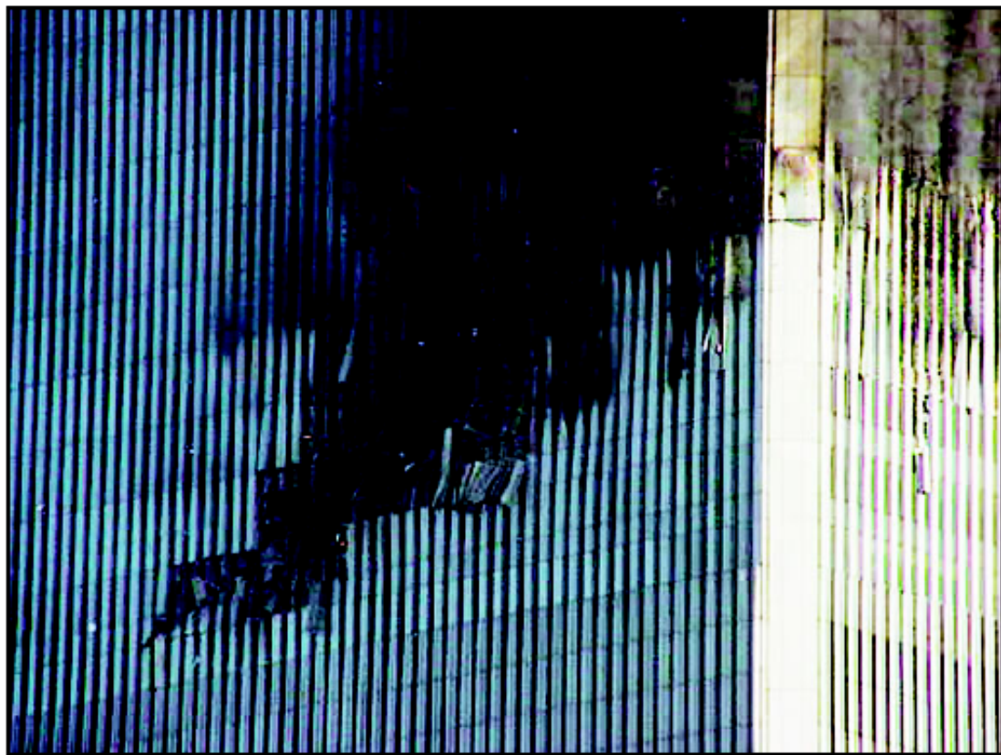
Porušení sloupů na záběru videokamery
