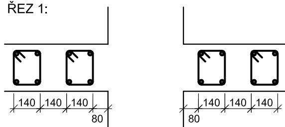
ŘEZ 1:
