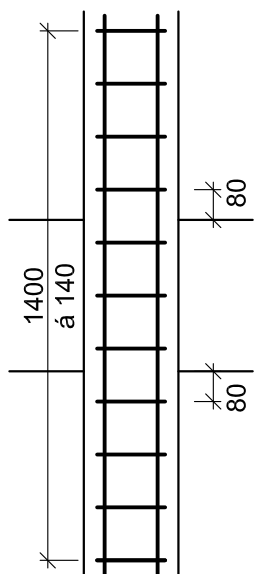
ŘEZ 2:
