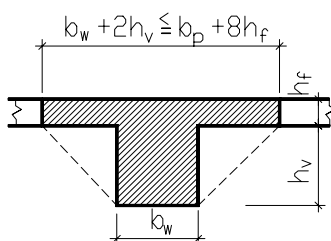
Obr. 1 Účinný průřez trámu ve směru vyšetřovaných momentů
