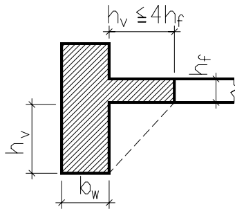
Obr. 2: Účinný průřez okrajového trámu
