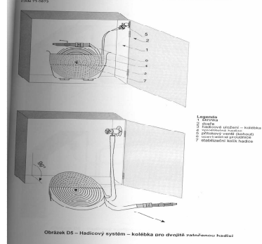
Obrázek D5 – Hadicový systém – kolébka pro dvojitě zatvárnou hadici
