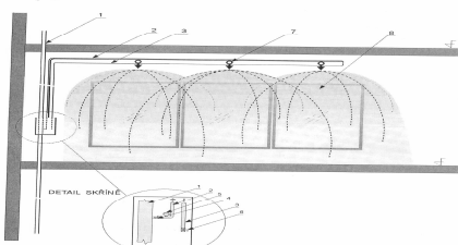
Obrázek D8 – Schéma provedení zkrápěcího zařízení
