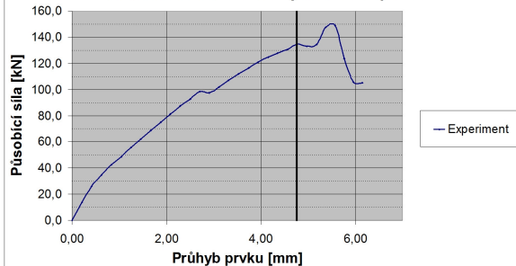
Zatěžovací křivka silně vyztuženého prvku
