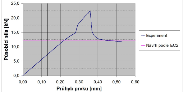
Zatěžovací křivka slabě vyztuženého prvku
