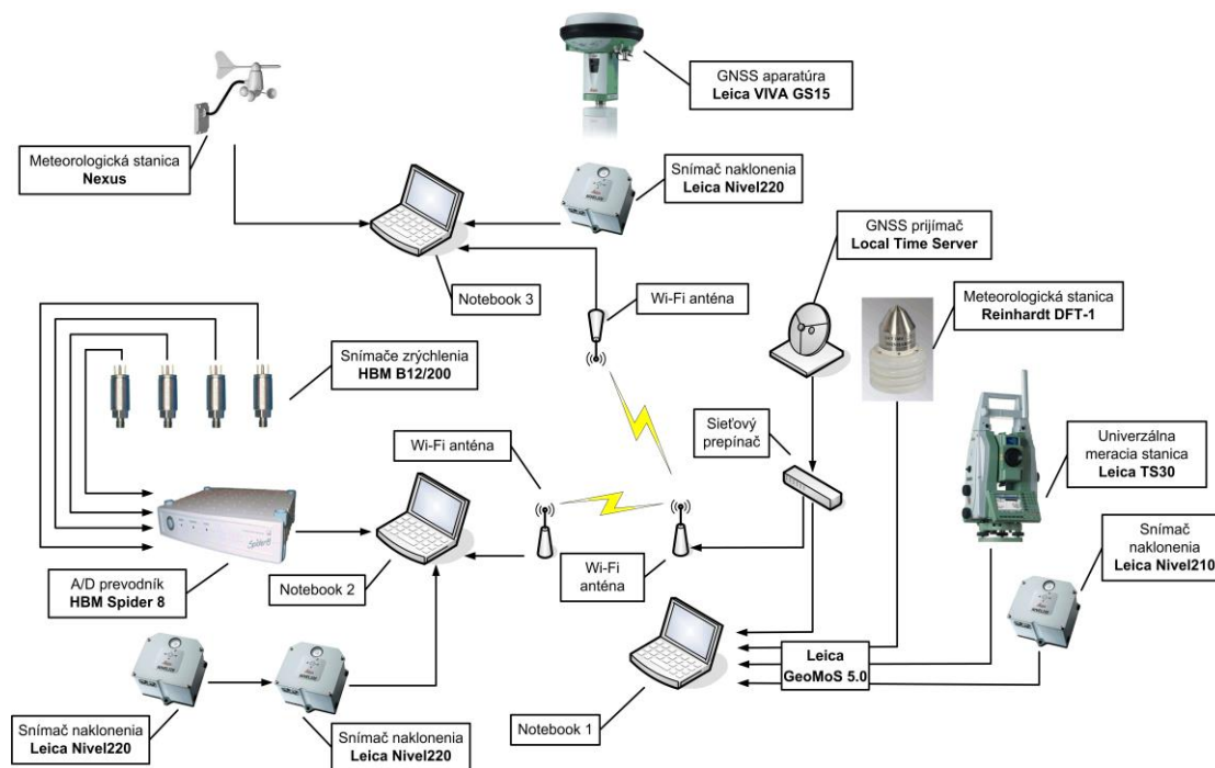
Obr. 1 Příklad schémy zapojenia komponentov AMS s časovou synchronizáciou
